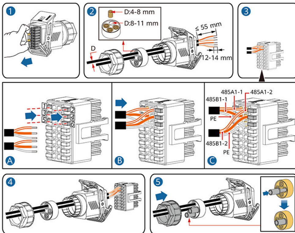
Abbildung 5-21 Kabelmontage
