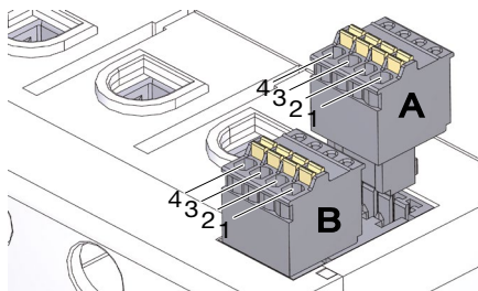
RS485-pistiku ühendusskeem:
