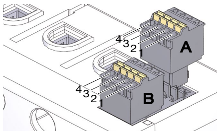
Anschlussbelegung des RS485-Steckers:
