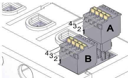
Διάταξη συνδέσεων βύσματος RS485:
